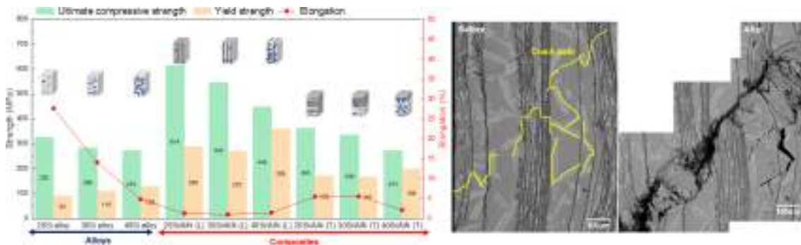
Fig. 4. (a) Al-Si 합금 및 Al-Si/AlN 복합재의 압축 특성 (b) Al-Si/AlN 복합재의 파단 특성
