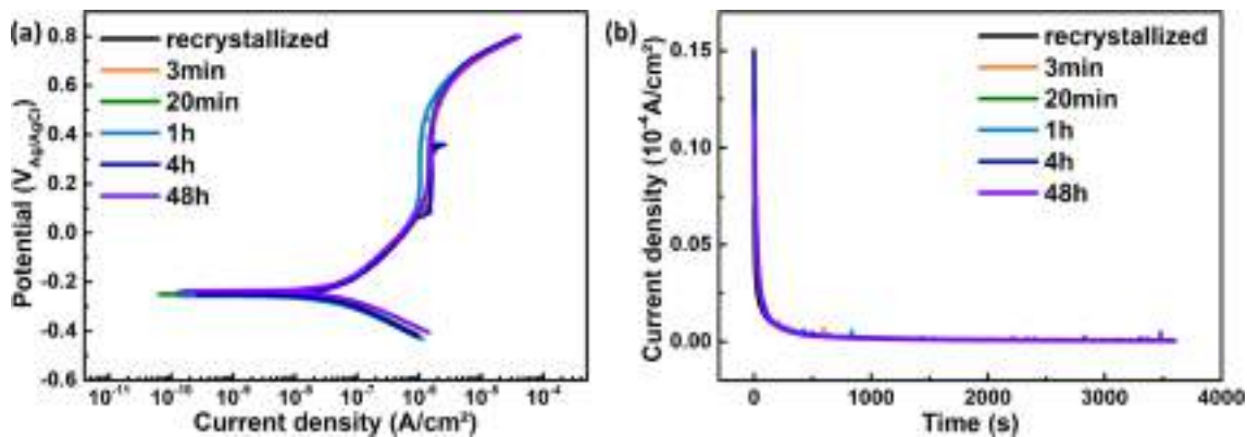
Fig. 1. (CoCrNi) 94 Al 3 Ti 3 (at.%) 합금의 열처리 시간에 따른 (a) 동전위 (b) 정전위 분극 거동의 변화
