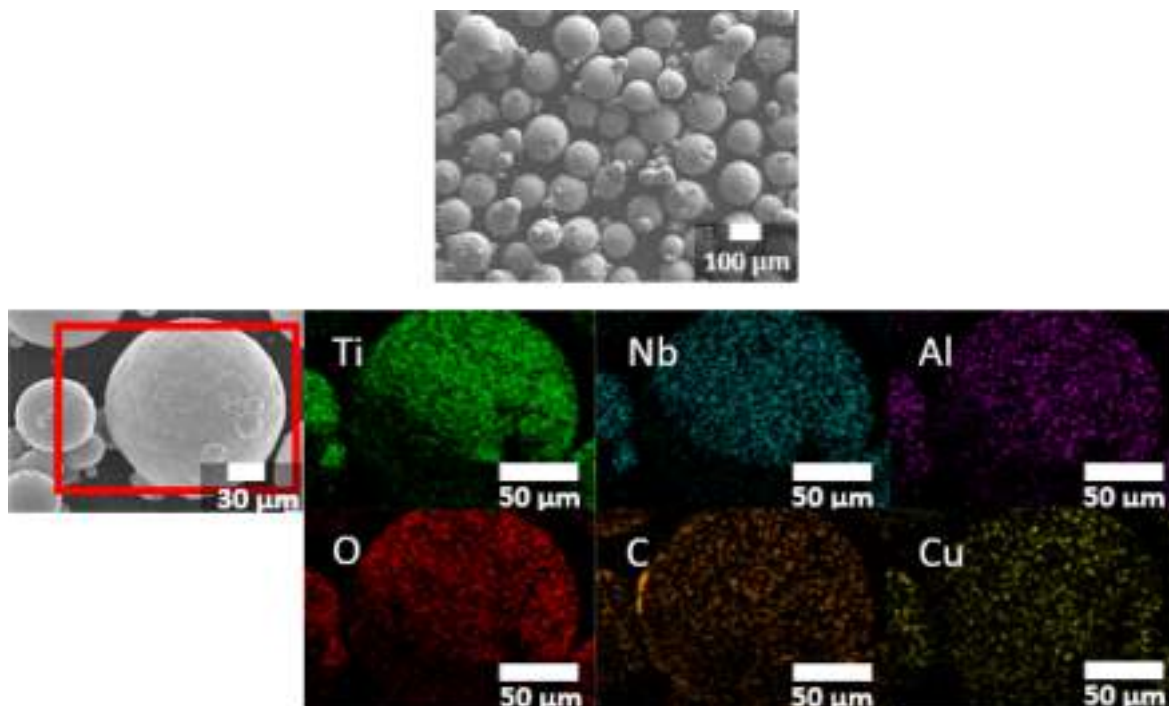
Fig. 1. (a) Atomized Ti-Nb-Al powder의 SEM-EDS 이미지
