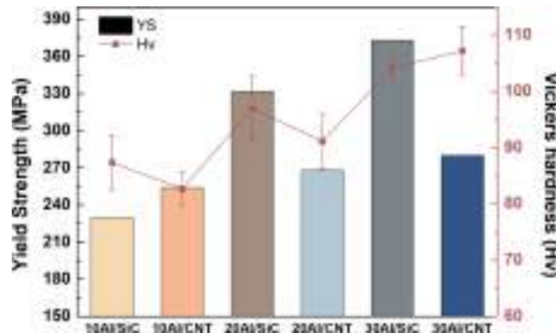
Fig. 1. (a) 순수 Al 기지, (b) Al6061 기지 복합재의 나노분말 종류 및 함량에 따른 항복강도와 비커스 경도 변화.
