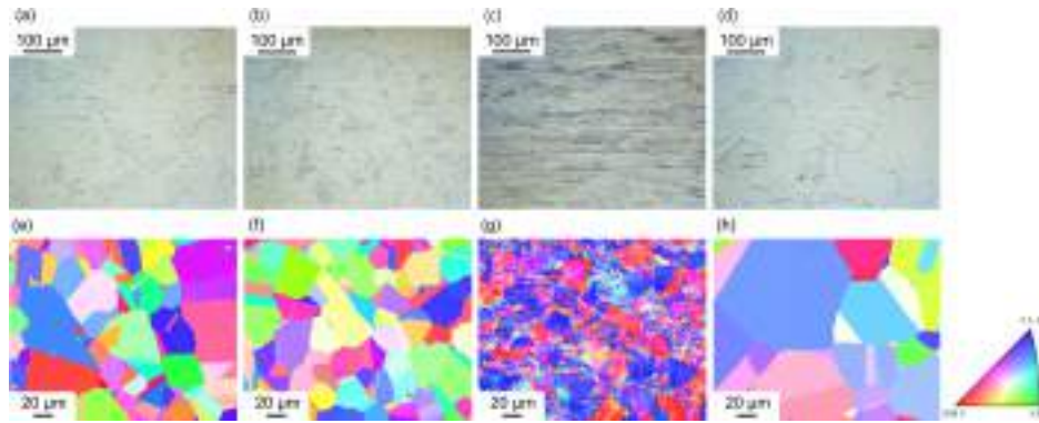
Fig. 1. 각 공정별 시편의 광학현미경 미세조직 이미지 (a ~ d) 및 IPF map 이미지 (e ~ f) (a, e: Forging, b, f: Hot piercing, c, g: Cold pilgering, d, h: Heat treatment)
