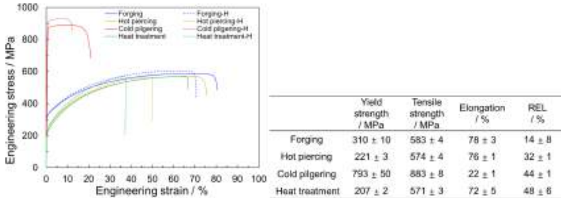
Fig. 2. 각 공정별 시편의 수소 장입 전(-)과 후(H)의 인장 곡선 및 수소 미장입 시편의 기계적 물성값
