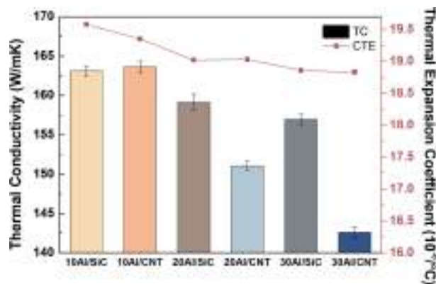
Fig. 2. 순수 Al 기지 복합재의 나노분말 종류 및 함량에 따른 열전도도 및 열팽창계수 변화.
