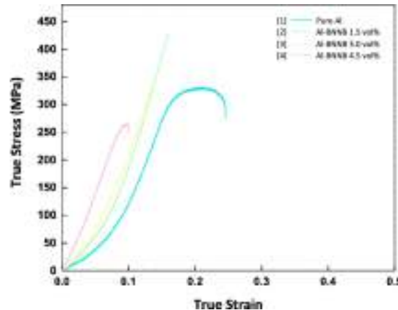
Fig. 2. Pure Al 및 Al-BNNB 복합재의 BNNB 함량에 따른 응력-변형률 곡선
