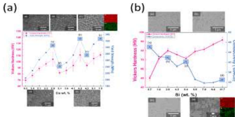
Fig. 3. (a)Cu, (b)Si 함량에 따른 경도, 항복 강도, 전기전도도 그래프>
