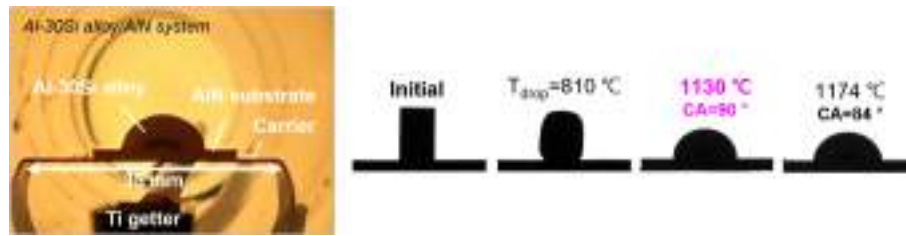
Fig. 1. Al-30Si 합금 - AlN 간의 젖음성 평가 결과
