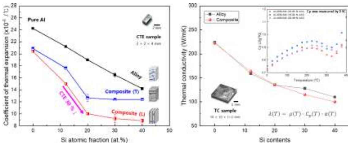
Fig. 3. (a) Al-Si/AlN의 열팽창 특성 (b) 열전도 특성
