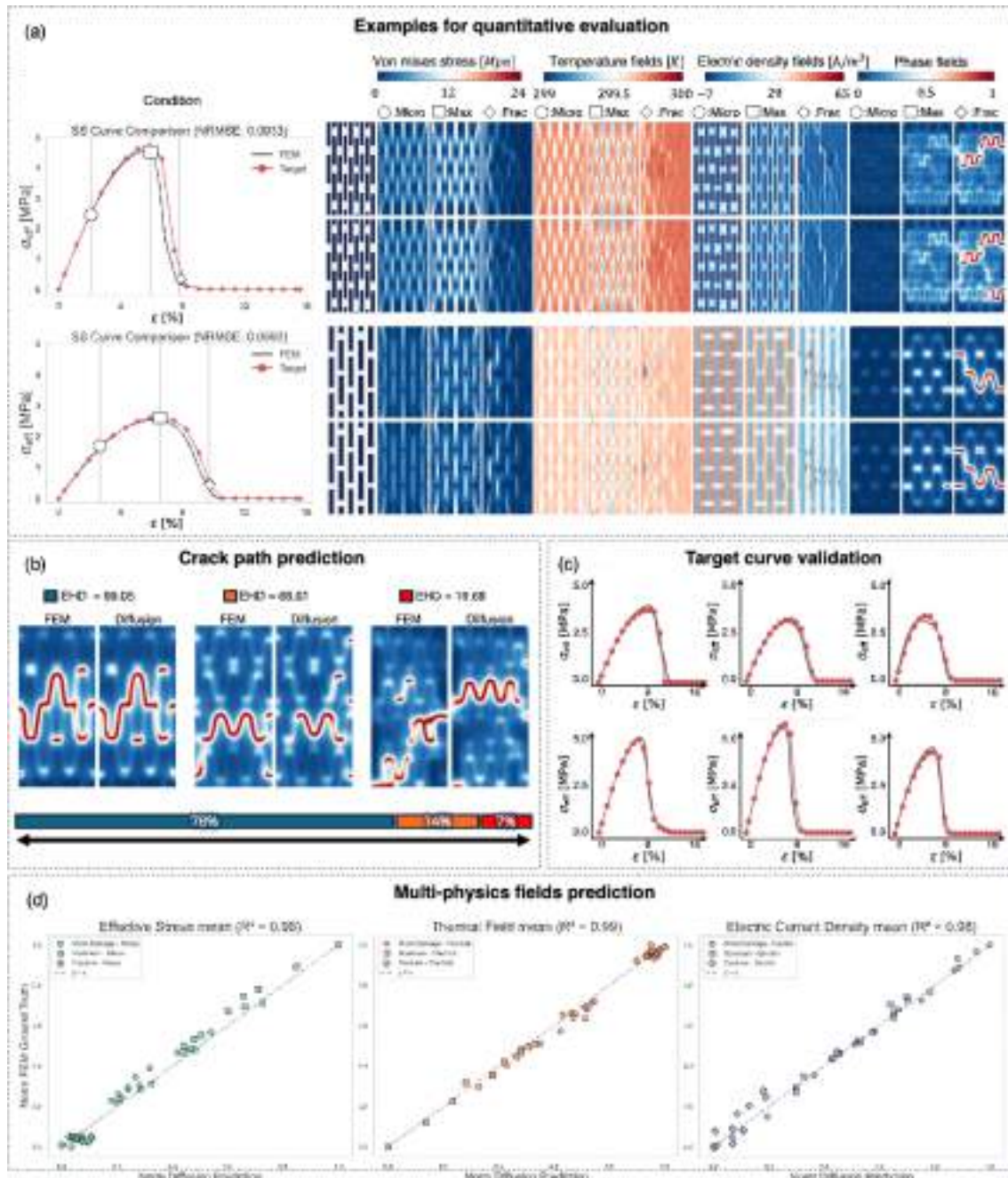
Fig. 2. FEM을 통한 Diffusion model의 validation 결과
