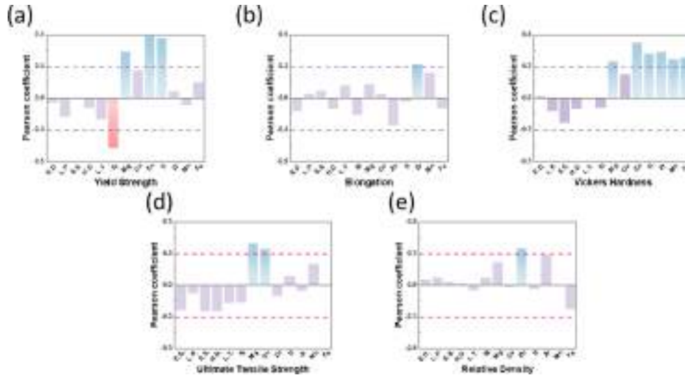
Fig. 2. 문헌 데이터의 공정 조건과 물성의 피어슨 상관 계수
