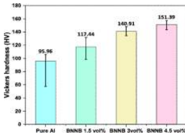
Fig. 1. BNNB 함량에 따른 Pure Al 및 Al-BNNB 복합재의 비커스 경도 변화
