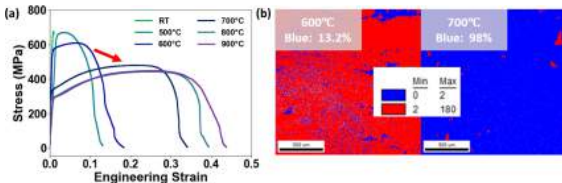
Fig. 1. Fe 64 Ni 36 (wt.%) 합금의 (a)열처리 온도에 따른 Stress-strain curves, (b)600°C 및 700°C에서 10분간 열처리한 시편의 EBSD-GOS map (Red: 변형된 영역, Blue: 재결정화된 영역)
