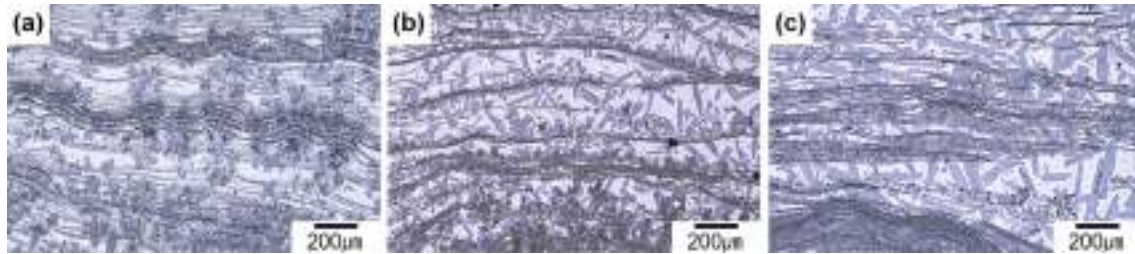
Fig. 2. Si 함량에 따른 복합재의 미세구조 (a) Al-20Si/AlN (b) Al-30Si/AlN (c) Al-40Si/AlN
